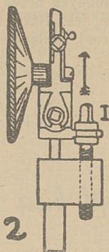
2 Przy strzale, który padł nisko: stawidło I wykreć.
