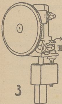
3 Przy strzale, który padł w prawo: stawidło II na prawo kręcić.
