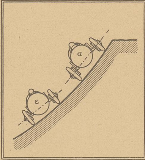
Rys. 134. Samochody na przewyższeniu toru. (Szybszy samochód nie może minąć samoch., a gdy nie mogąc wzniesić się wyżej na przewyższenie przy zwiększonej szybkości, ulegnie poślizgowi (zarzuceniu) ku środkowi krzywizny). Mijanie się na torze z lewej strony.
