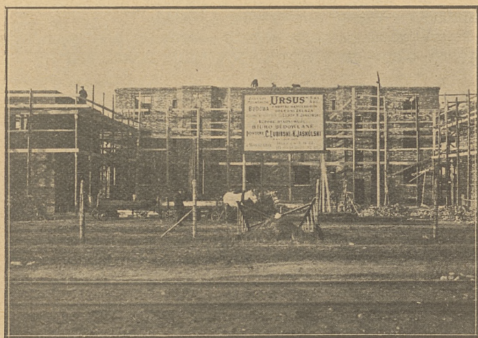
Rys. 218. Widok fabryki od strony toru kolejowego.
