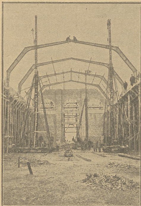
Rys. 215. Budowa odlewni.
