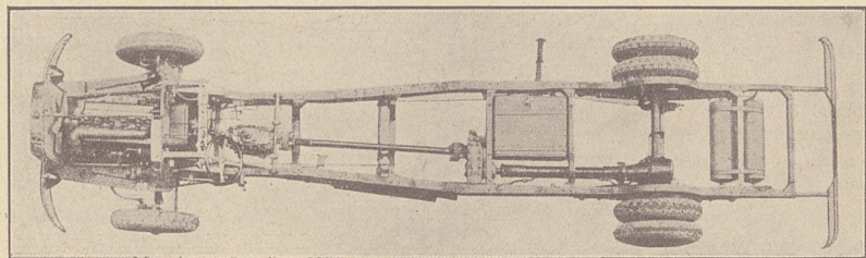
Autobusowe podwozie Magirus.
