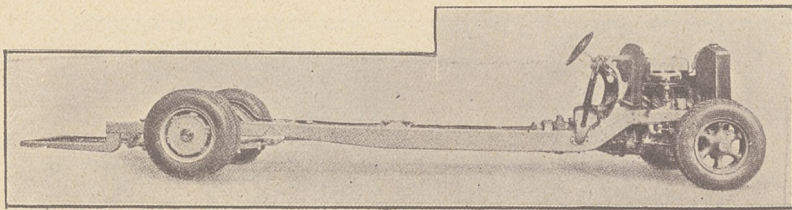
Autobusowe podwozie M. A. N.
