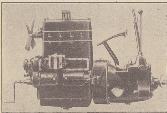
Silnik szybkiego podwozia Laffly,
