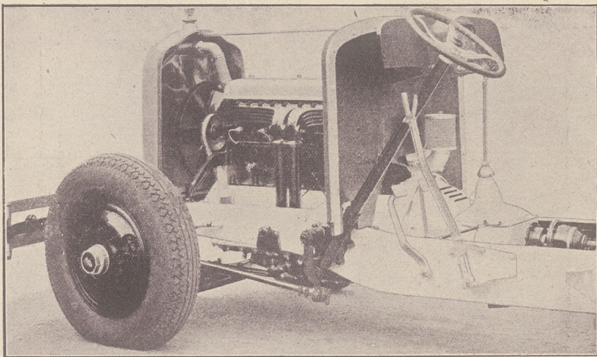
Przód podwozia autobusowego White.
