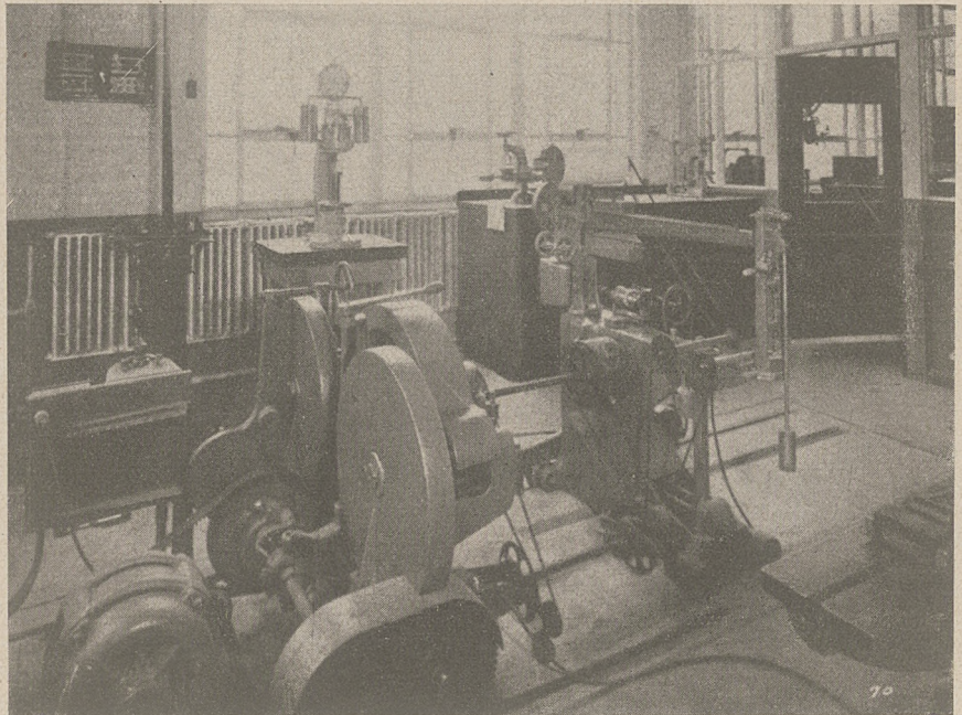
Torsjonomierz, przyrząd notujący kąt skręcenia i punkt przelamania wałów.
