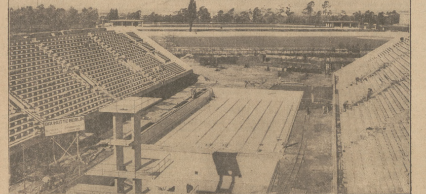
OLIMPIJSKI BAZEN PŁYWACKI W BERLINIE znajduje się w stadium wykańczania i przedstawia się już dziś w imponujący sposób.
