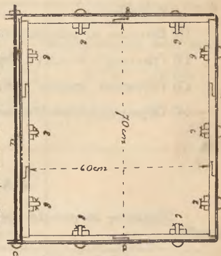
Szafka złożona Przekrój A—B
