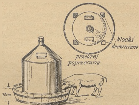
Ryc. 13. Praktyczne poidło dla prosiąt.
