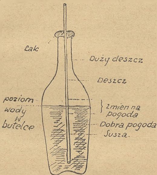
Ryc. 6. Tani barometr.
