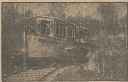
Nasza rycina przedstawia łódź motorową zaopatrzoną w koła. Motor łodzi, który na wodzie porusza jej propeller, gdy łódź dobiła do brzozy, porusza na lądzie jej koła i wprawia ją w ruch. Na rycinie widzimy ten motor, gdy łódź ląduje i wjeżdża na szyny. Po obu stronach brzozy znajduje się urządzenie, które wyciągnąwszy łódź z wody, ustawia ją na szynach.
