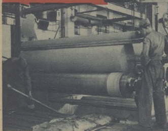
Uczeń S. P. P. zajęty naprężaniem filtrów suszących.
