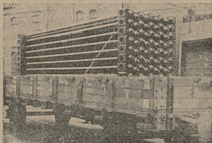
Transport sekcji wężykowatych do kotłów selekcyjnych wysokoprężnych
