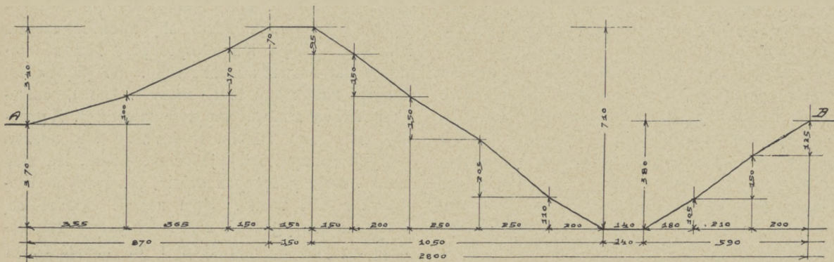
PRZEKRÓJ GÓRY ZAMKOWEJ W CIESZYNIE.
