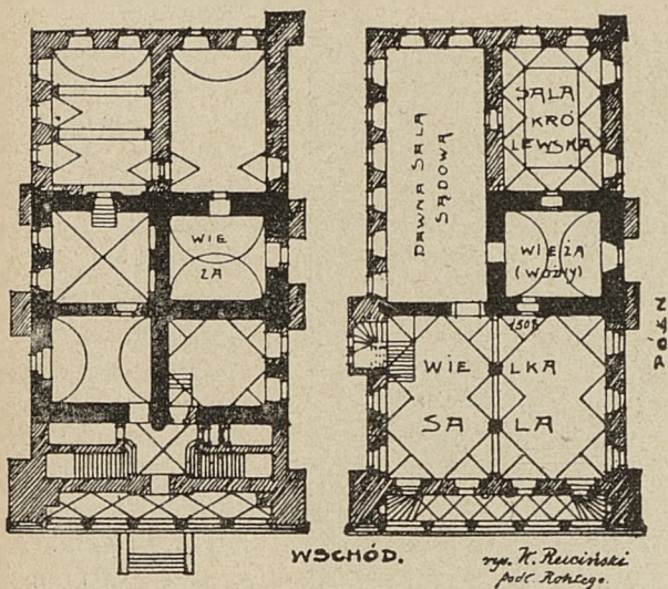
Rzut poziomy ratusza poznańskiego Sk. — 1 : 400
