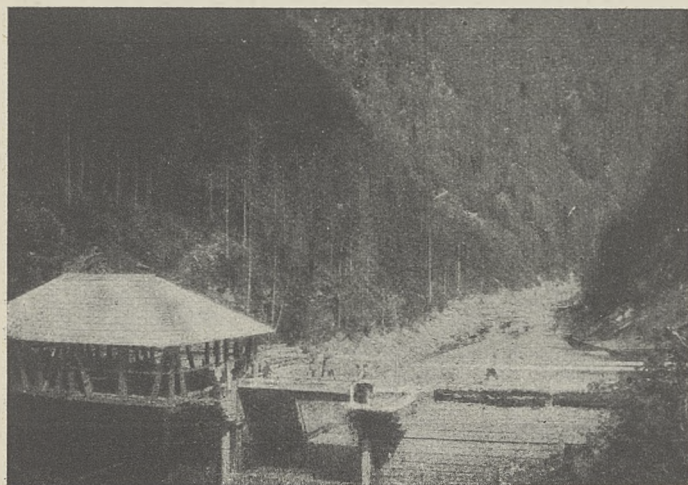
Ryc. 235. KLUZA „MARIEN” Fot. inż. W. Chudzikiewicz. PRZY UJŚCIU POTOKU MARIEN DO CZEREMOSZU BIAŁEGO.
