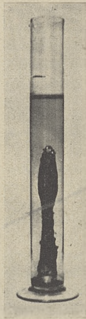
Ryc. 237. Grot żel. w paskach cynkowych po 24 godz. działaniu roztworu sody żrącej.
