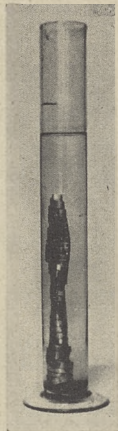
Ryc. 230. Grot żel. w paskach blachy cynkowej w roztworze sody żrącej.
