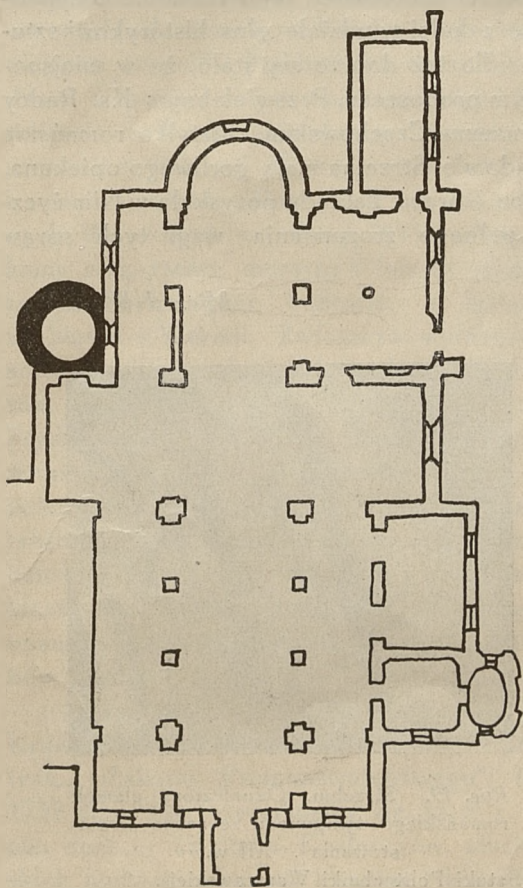
Ryc. 15. Strzelno. Plan bazyliki z uwidocznieniem fundamentami odkopanej baszty romańskiej.
