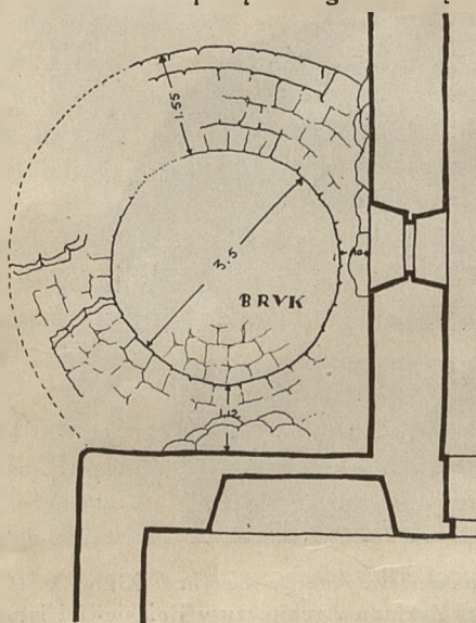
Ryc. 16. Strzelno. Rzut poziomy odkopanej baszty.
