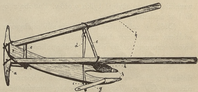
Ryc. 244. Socha łopatkowa. (Mieczysławów. pow. postawski, Muzeum U. S. B. Wilno. Rys. własny). a—rogał, b—obże, c—poprzeczka, d—powój, e—klin, f—narogi, g—prypolek, h—łopatka (polica) i—podsosznik.
