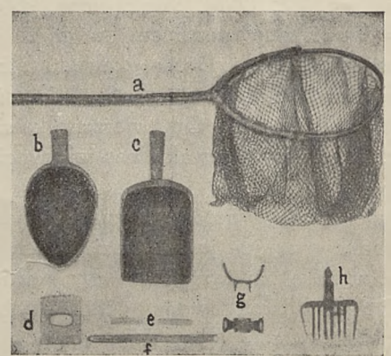
Ryc. 231. Fot. M. Znamierowska-Prüfferowa. Pomocnicze sprzęty rybackie z okolic Mężenina n/B. a—koszorek, b—korczak, c—szufelka, d, e—kłódki, f—kleszczka, g—chrapię, h—ości
