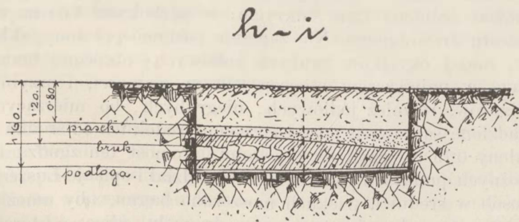
Fig. 4. Przekrój pionowy wykopu E z fig. 1, po linii h—i (Skala 1:100).
