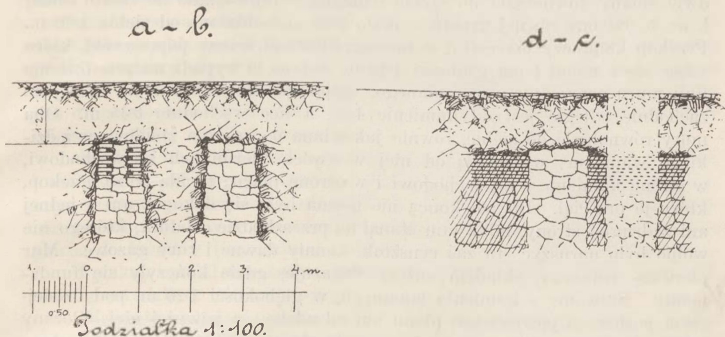
Fig. 3. Przekrój pionowy muru D po linii a—b oraz d—c .
