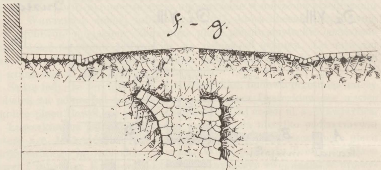
Fig. 2. Przekrój pionowy po linii f—g . (Skala 1: 100).
