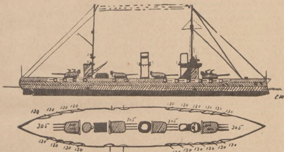
Лінійний корабель-дреднаут „Воло“ 1914 р., 23.000 тон. 21,6 вуз. 12—12 дм., 20—130 мм., 4—75 мм. протилітакових гармат, 4 кулети, 4 підводних міних апарати. Випах на 1 борт 4.100 кг. Екіпаж 42 старшин і 1200 морців.
