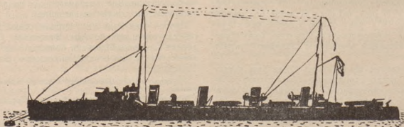
Ескадринний міноносець „Завидний“ (1903 р. в Миколаїв) С.Ш. 400 тонн, 27 вузлів; 2 гармати 15 см 4 кулемети 2 міни обидві - 4 Сторожки і 60 мінарів.
