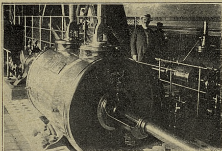
Główna maszyna parowa.
